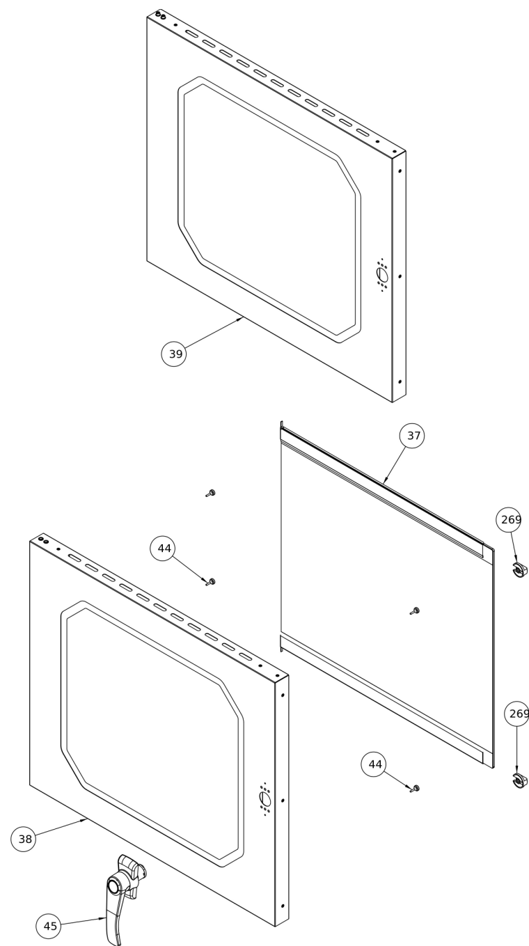
Door
